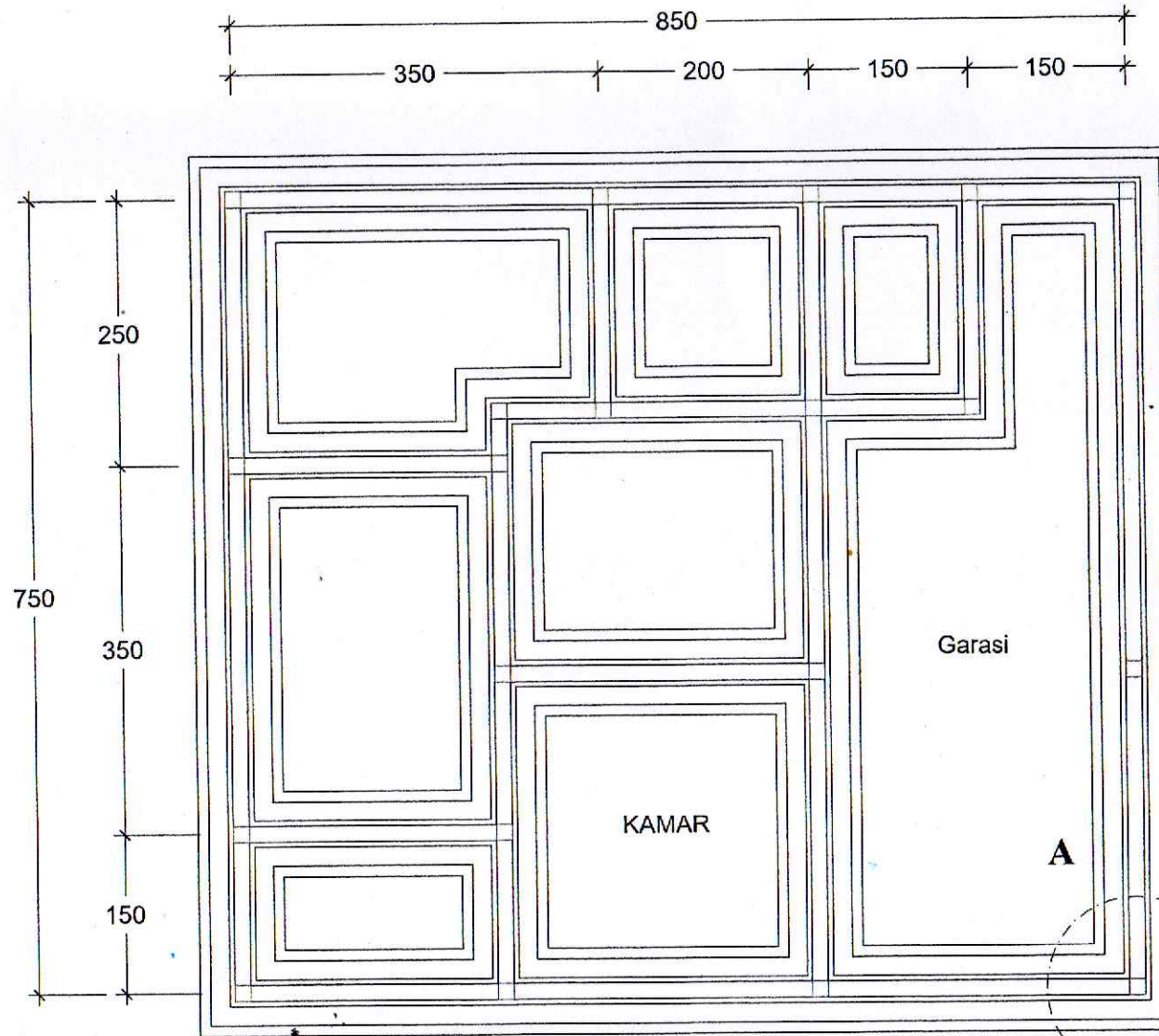
DENAH PONDASI
