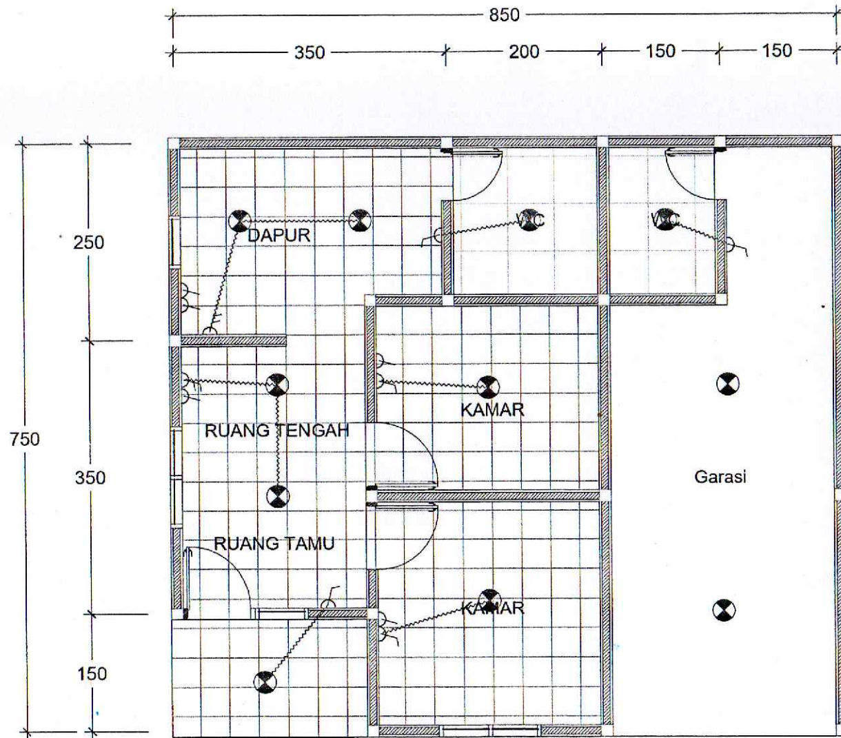
DENAH KELISTRIKAN
