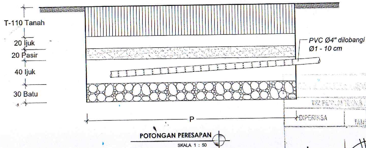
Dimensi Peresapan
