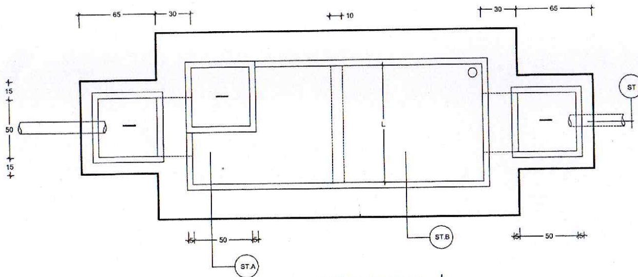
DENAH SEPTIKTANK
