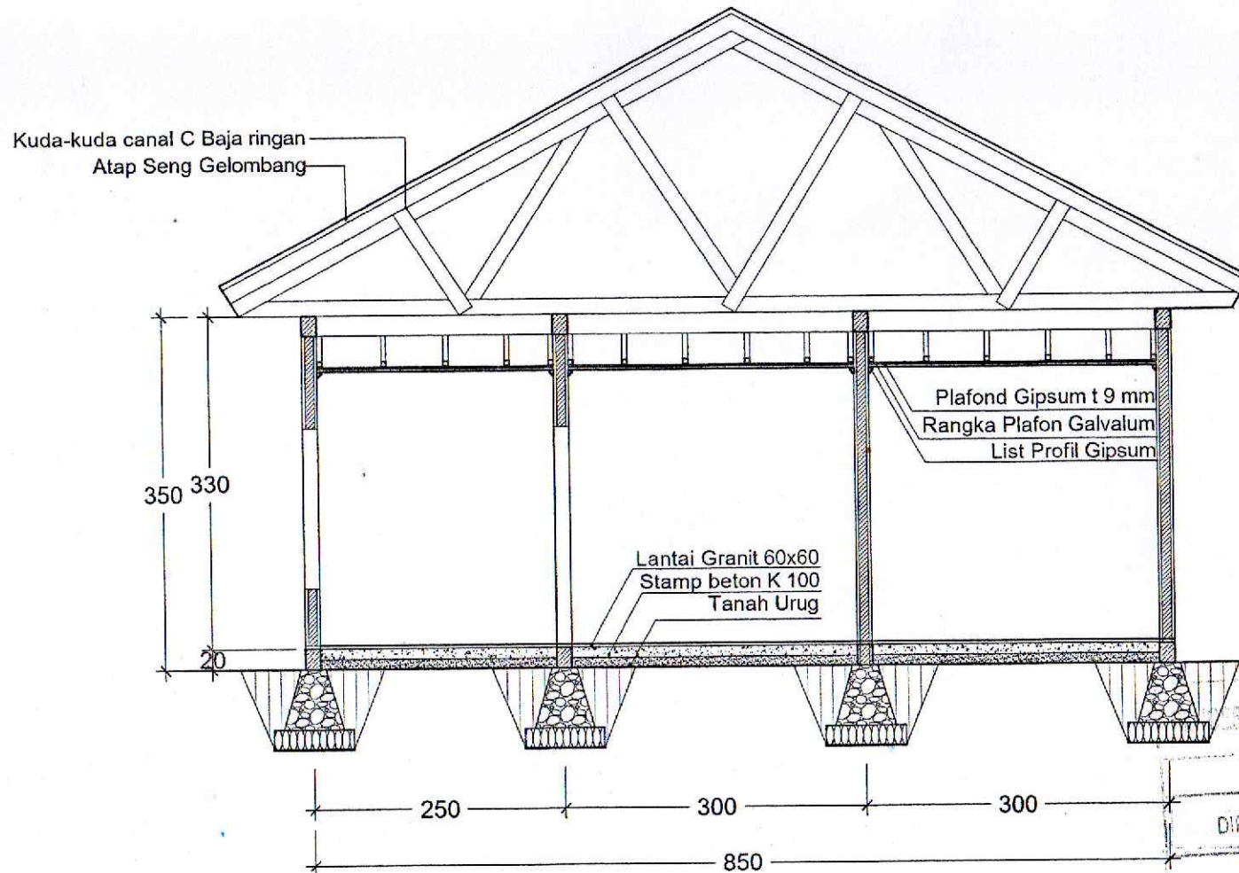
POTONGAN MELINTANG (A-A)
